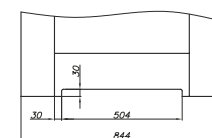
skrzydło „80” z podcięciem wentylacyjnym
