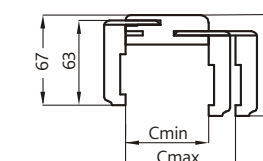
Przekrój TUN
