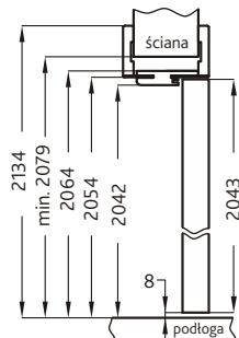
Przekrój pionowy drzwi bezprzylgowych ORB
