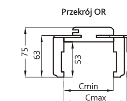
Przekrój pionowy drzwi przylgowych
