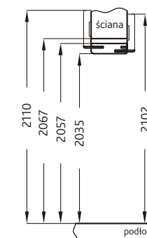
Wymagana szerokość otworu w murze 2067 mm
