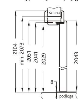
Wymagana wysokość otworu w murze 2073 mm
