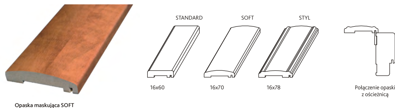
Opaska maskująca SOFT
