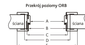
D - wymagana szerokość otworu w murze
