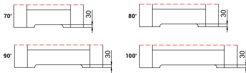
Wielkość podcięcia wentylacyjnego w drzwiach ramowo-płycinowych w zależności od szerokości skrzydeł drzwiowych **)
