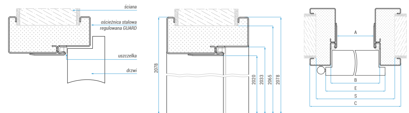
▼ OŚCIEŻNICA GUARD STALOWA REGULOWANA
