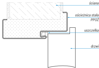
▼ OŚCIEŻNICA PPOŻ STALOWA STAŁA
