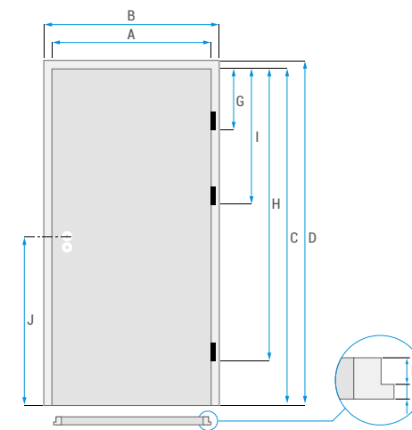
Wymiary skrzydeł drzwiowych przylgowych:
