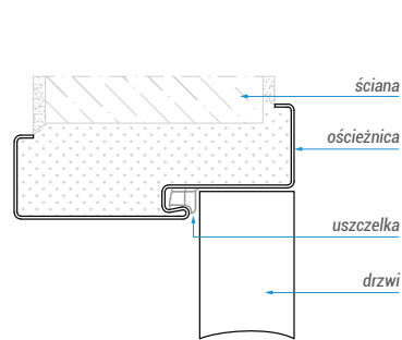
▲ OŚCIEŻNICA STALOWĄ STALOWĄ BEZPRZYLGOWĄ
