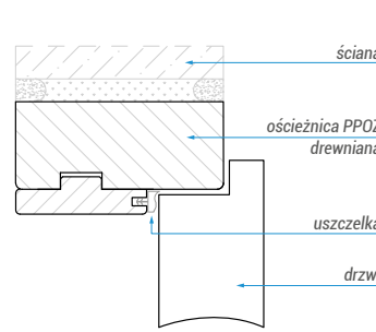
▲ OŚCIEŻNICA PPOŻ DREWNIANA
