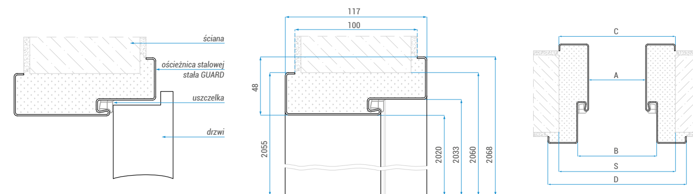
▲ OŚCIEŻNICA GUARD STALOWA STAŁA
