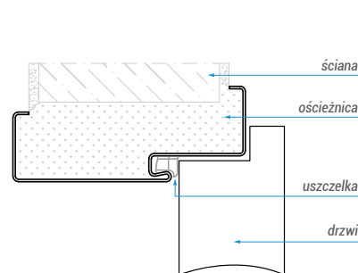
▼ OŚCIEŻNICA STALOWĄ STALOWĄ
