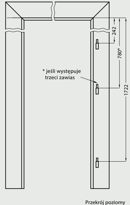
Przekrój ościeżnicy regulowanej TOP
