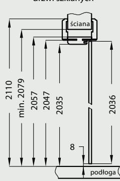
Przekrój pionowy drzwi szklanych
