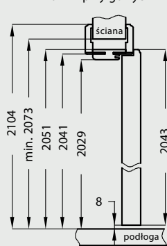
Przekrój pionowy drzwi przylgowych
