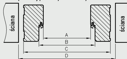
przekrój poziomy ościeznicy w murze
