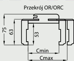
Przekrój pionowy drzwi przylgowych
