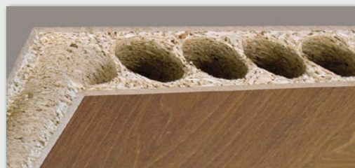
Rys.B. Płyta wiórowo-otworowa
